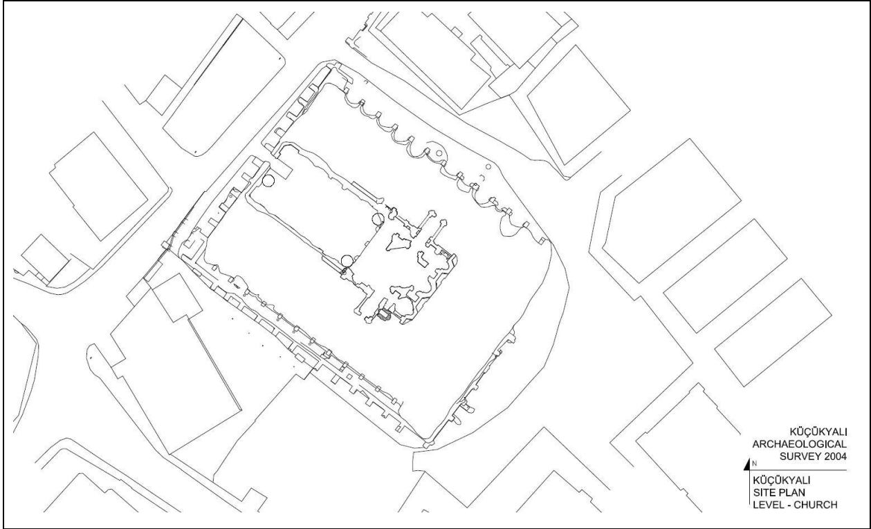
Şekil 5: Küçükalyı'daki arkeolojik alanın 2004 yılında hazırlanan vaziyet planı (KYAP Arşivi, 2004)
