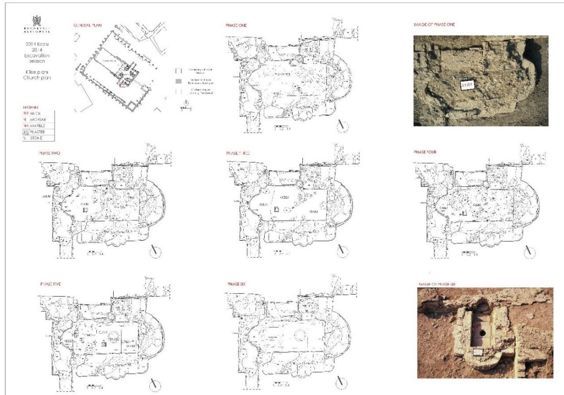
Şekil 2: Kilisenin güneydoğusuna eklenen mezar şapelinin kazı evreleri; mezar şapelinin yeri genel planda görülmektedir (KYAP Arşivi, 2015)
