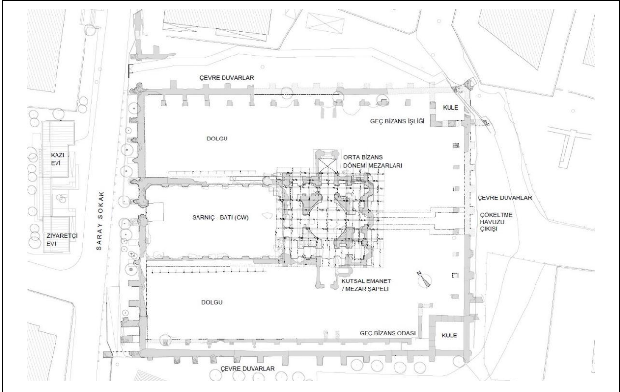
Şekil 4: Küçükaly'daki arkeolojik alanın mevcut vaziyet planı (KYAP Arşivi, 2019)
