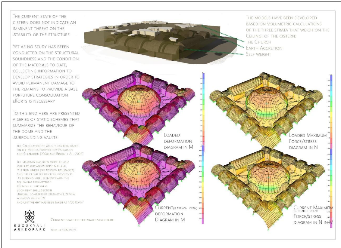
Şekil 10: 2016 yılında Doğu Sarnıç üst örtü analizleri (KYAP Arşivi, 2016)
