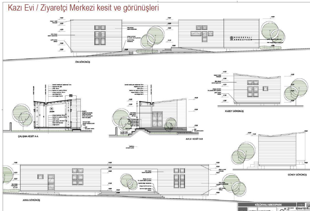
Şekil 18: Küçükyalı kazı evi ve ziyaretçi merkezi projesi (KYAP Arşivi, 2015, Atölye Mimarlık tarafından 5 Numaralı Kültür Varlıklarını Koruma Bölge Kurulu'nun onayına sunulmuş ve Mayıs 2015 tarihinde onaylanmıştır.)
