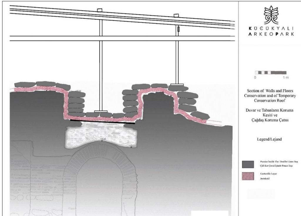
Şekil 15: 2017 yılında geçici çatının katmanlarının iyileştirilmesi (KYAP Arşivi, 2017)
