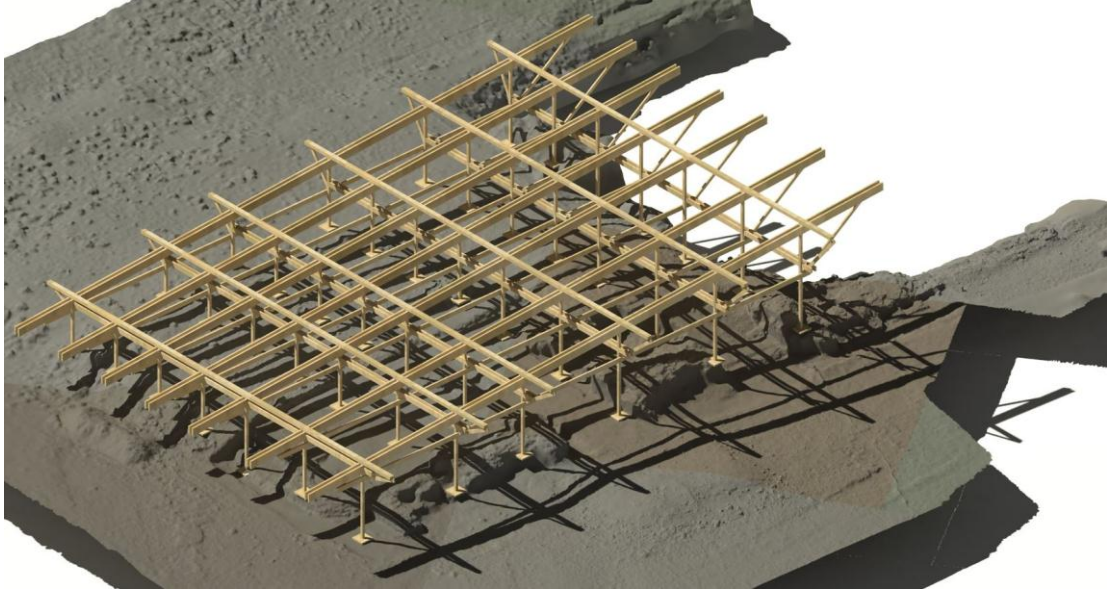
Şekil 8: 2016 yılında Mimar M.S. Bermek tarafından tasarlanan ilk koruma çatısı (KYAP Arşivi, 2016)
